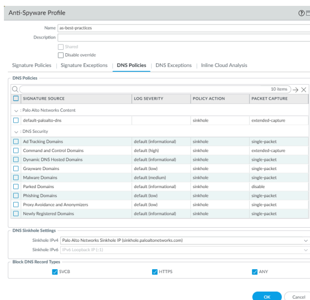
Figure 3: Políticas DNS de perfiles de antispyware
