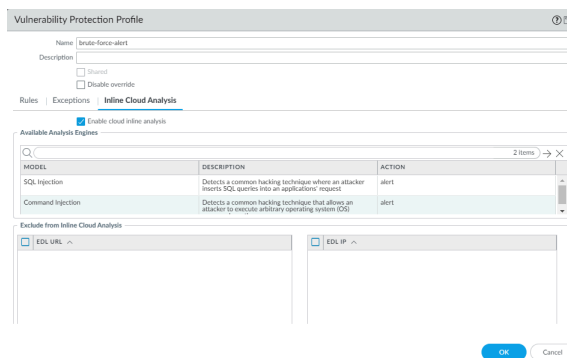
Figure 2: Análisis en línea en la nube alerta el perfil de protección frente a vulnerabilidades
