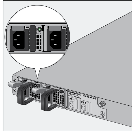
Входы питания PA-850
