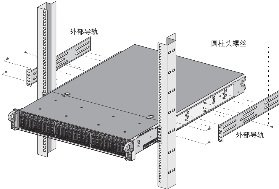
图 9. 安装外部导轨完成后将机箱固定到机架
