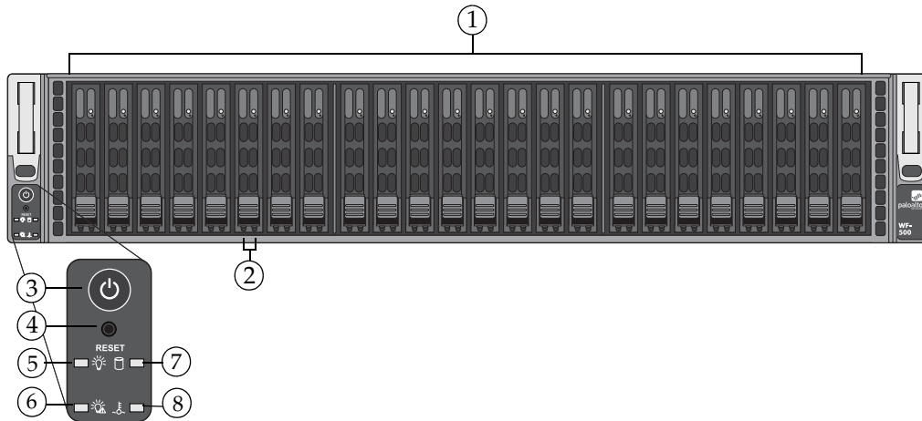
图 1. 前面板
