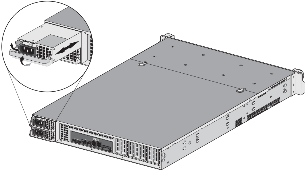
图 13. 电源更换
