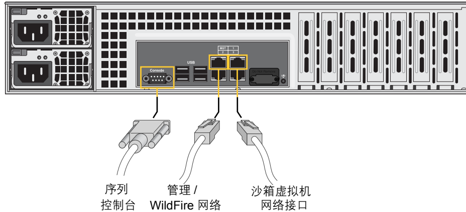
图 10. WF-500 设备背面的电缆连接
