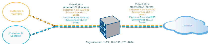
圖 1: 含子介面的虛擬交接部署 (僅 VLAN 標籤)
